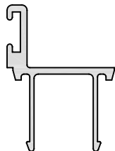
PAR 107 35mm DOOR STOP A/P: 135.28 mm L/W: 0.210 kg/m
