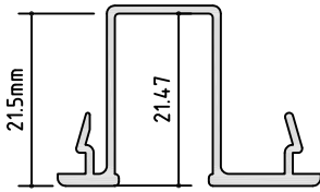
PM 755 SCREEN ADAPTOR A/P: 184.12 mm L/W: 0.276 kg/m
