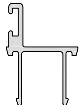
PAR 111 38mm DOOR STOP A/P: 133.18 mm L/W: 0.210 kg/m
