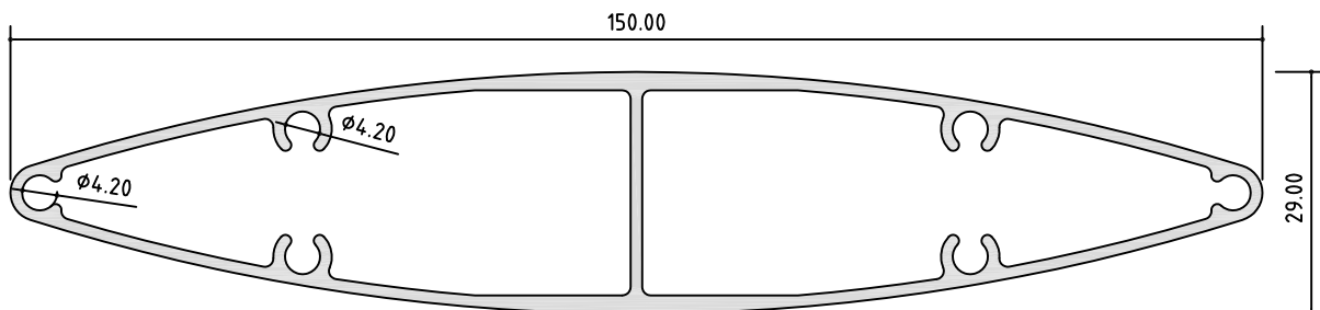
LVR20031 LOUVRE BLADE A/P: 312.32 mm L/W: 1.557 kg/m
