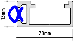
PM 722 UNIVERSAL DOOR STOP BASE A/P: 131.36 mm L/W: 0.255 kg/m
