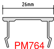
PM764 67mm DG POCKET FILLER A/P: 113.88 mm L/W: 0.185 kg/m
