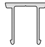
ME2-20230 POCKET FILLER A/P: 108.95 mm L/W: 0.186 kg/m
