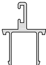
PAR 106 45mm DOOR STOP A/P: 133.18 mm L/W: 0.210 kg/m
