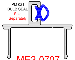
ME2-0707 45mm DOOR STOP A/P: 183.61 mm L/W: 0.386 kg/m
