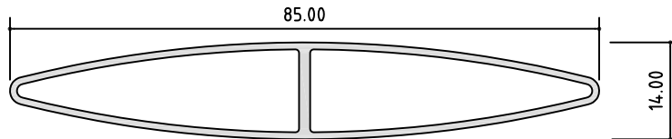
LVR51532 LOUVRE BLADE A/P: 176.21 mm L/W: 0.522 kg/m
