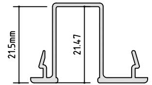
PM 755 SCREEN ADAPTOR A/P: 184.12 mm L/W: 0.276 kg/m
