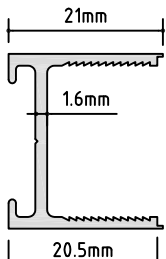
PM770 21mm L/W STILE A/P: 150.08 mm L/W: 0.265 kg/m
