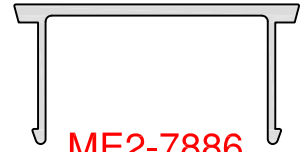
ME2-7886 DG POCKET INFILL A/P: 144.57 mm L/W: 0.277 kg/m
