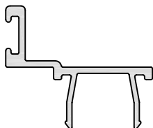
PAR 206 45mm DOOR STOP A/P: 132.19 mm L/W: 0.227 kg/m
