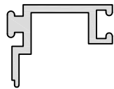
PM 828 SG ADAPTOR A/P: 98.53 mm L/W: 0.195 kg/m
