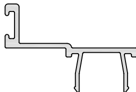
PAR 207 38mm DOOR STOP A/P: 146.19 mm L/W: 0.250 kg/m
